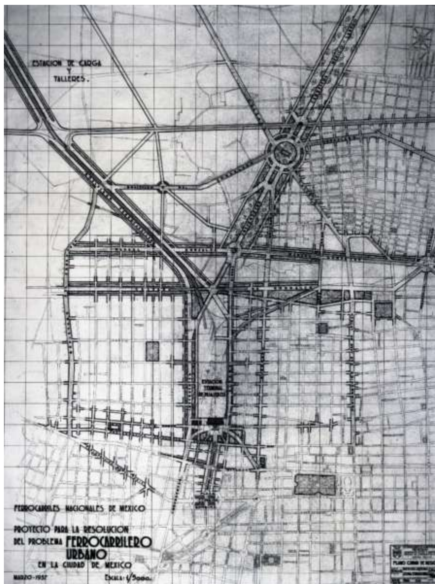
Plano del proyecto para la resolución del problema ferrocarrilero urbano en la ciudad de México. Marzo 12 de 1937. Zona de las estaciones. Fondo Ferrocarriles Nacionales de México. Sección Comisión de Avalúo e Inventarios. Secretaría de Cultura/CNPPCF/CEDIF.
